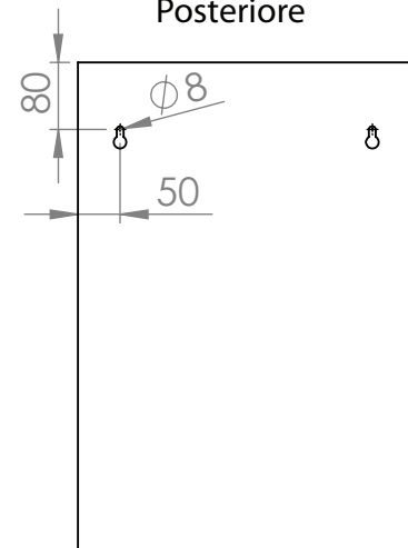
Posteriore
