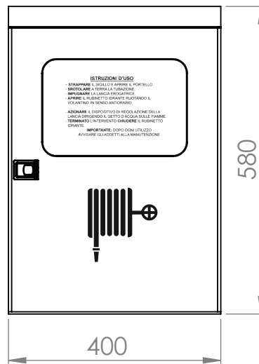
Frontale
