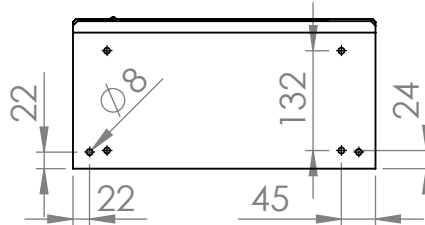
Frontale
